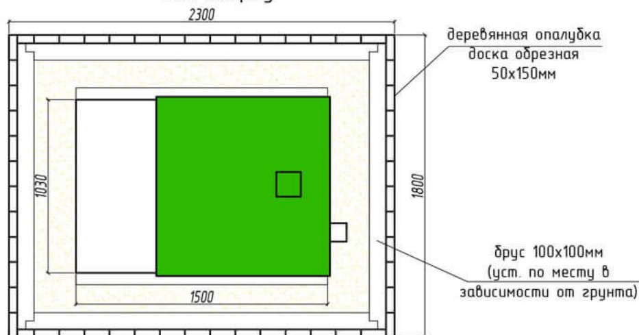
Вид сверху
