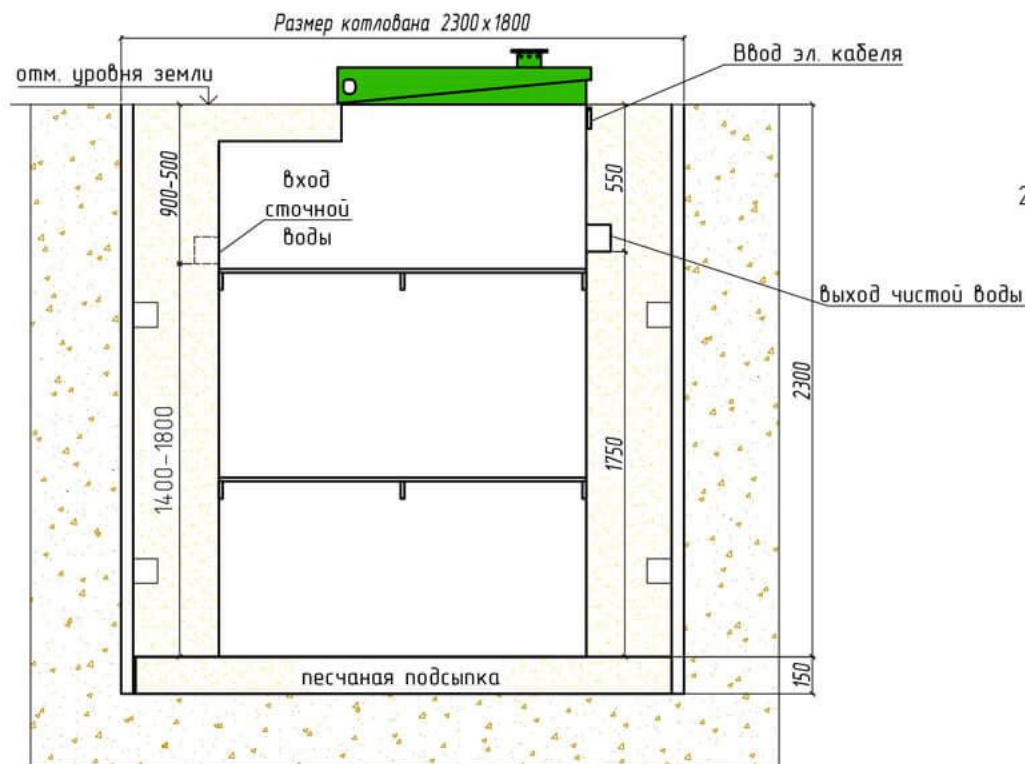
Вид сбоку
